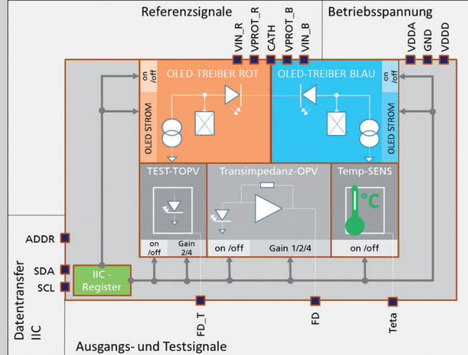
Blockschaltbild des Sensorchips
